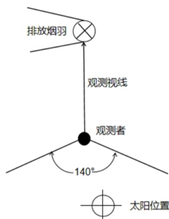
图2 观测视线与太阳位置示意图
